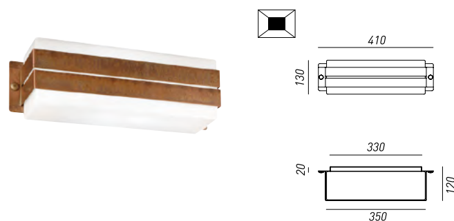
252.09.RR 252.09.RF 2x Max 30W E27 252.59.RR 252.59.RF LED 13W 3000K IP 54
