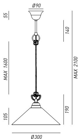
212.10.0V 2x Max 77W E27
