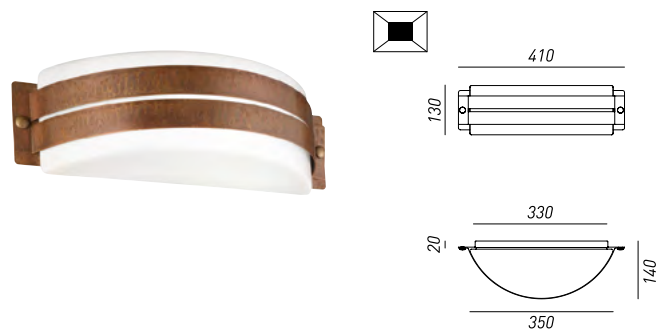
252.07.RR 252.07.RF 2x Max 30W E27 252.57.RR 252.57.RF LED 13W 3000K IP 54
