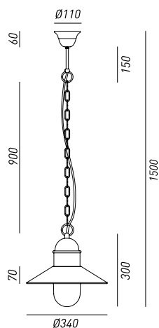
244.02.ORB 244.02.ORT 1x Max 57W E27 1x Max 23W E27 ES IP 43
